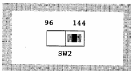
Fig. 2.2 Select 144 or 96 I/O
